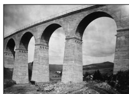
Wisła-Głębcze. Władukt kolejowy na dcinku Wisła- Dziechcinka – Wisła-Głębcze, zaprojektowany przez tandem inżynierski: Stefan Sasaki i Tadeusz Mejer, fot. J. Bułhak, 1936
